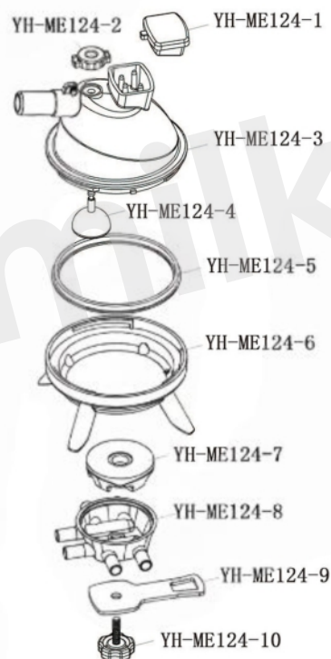
YH-ME124-7 Опорный блок YH-ME124-8 Распределитель воздуха YH-ME124-9 Ручка YH-ME124-10 Гайка
